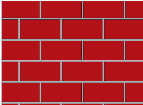
Половинная перевязка
